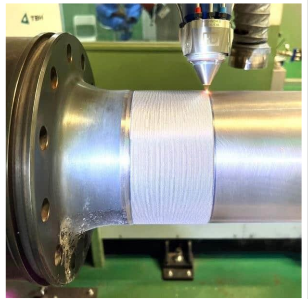
피스톤 로드 클래딩
