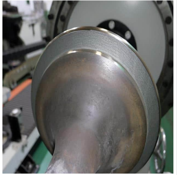
배기 밸브 스프indel 리드 표면 클래딩
