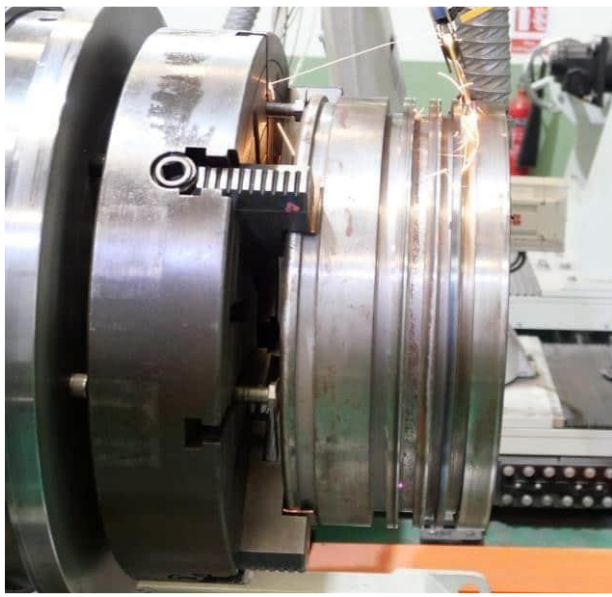
피스톤 링 홈 클래딩
