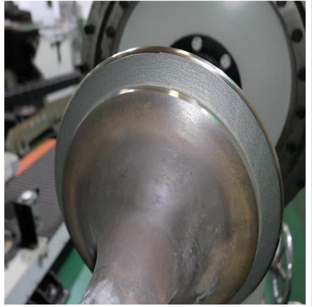
배기 밸브 스�핀들 리드 표면 클래딩
