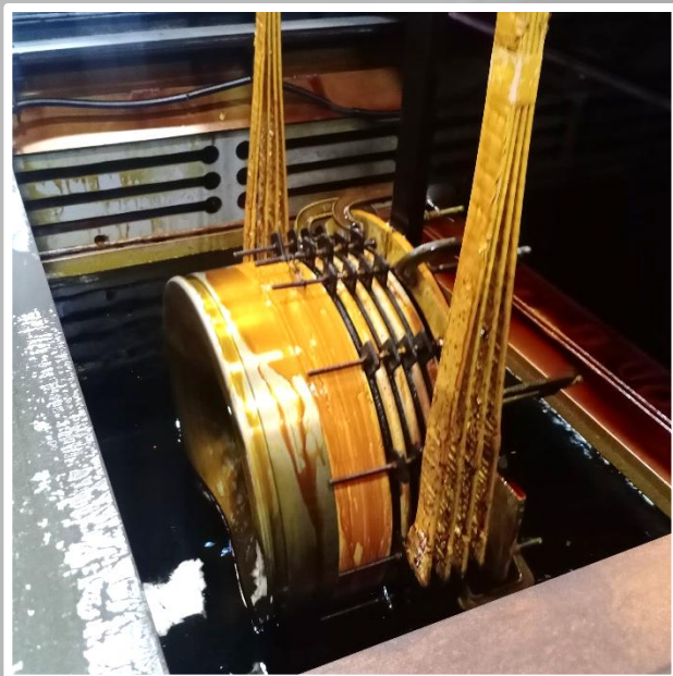
ピストンリング溝 硬質クロムメッキ加工
