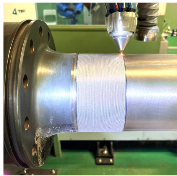
ピストンロッド
