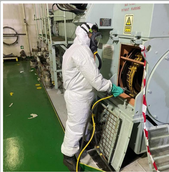
オルタネーターの化学洗浄
