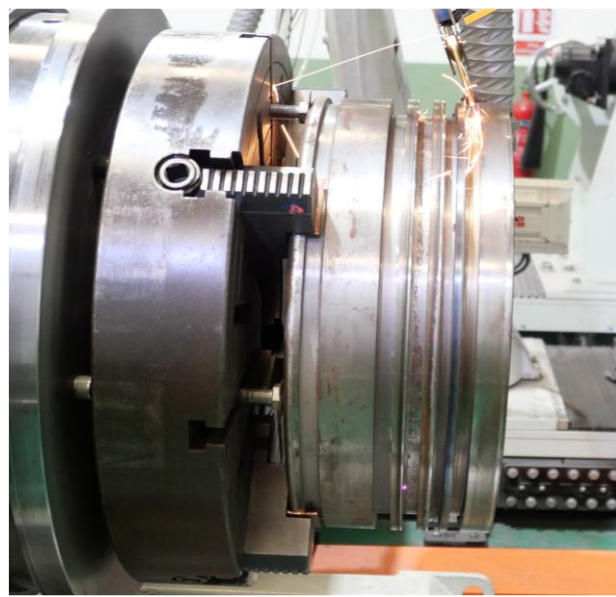
ピストンリング溝
