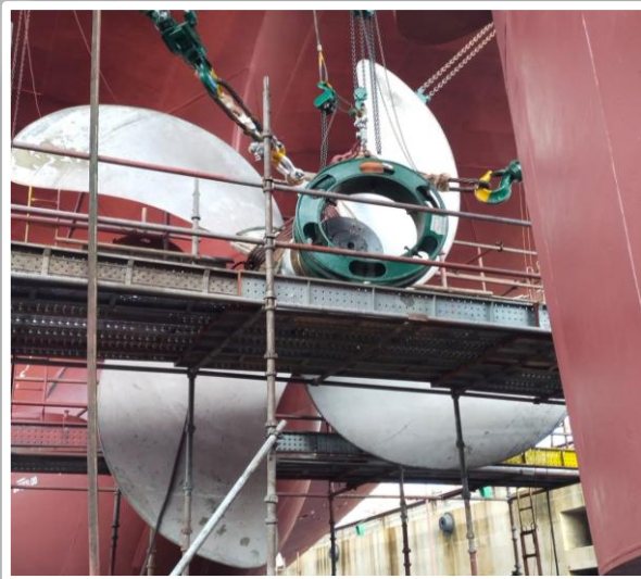
プロペラの取り付け
